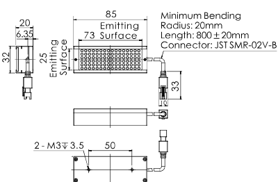
4.OPT-LI8532
