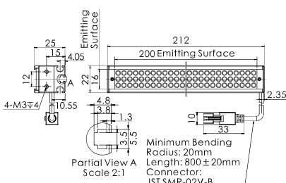
14.OPT-LI21222
