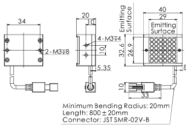
1.OPT-LI4033
