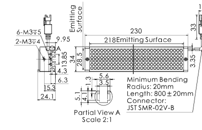
15.OPT-LI23034
