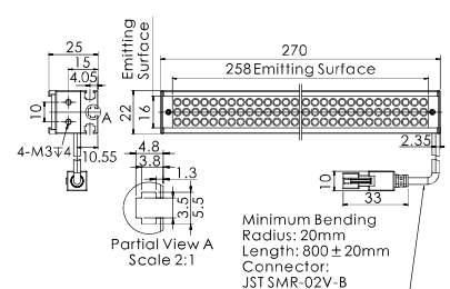
17.OPT-LI27022
