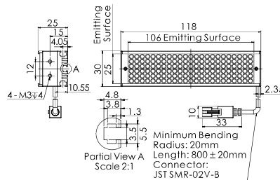
8.OPT-LI11830
