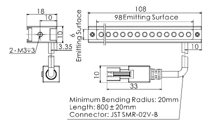
9.OPT-LI14030
