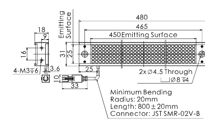
21.OPT-LI48031
