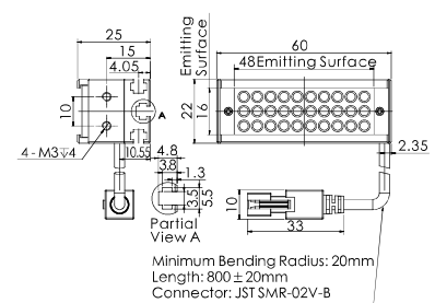
3.OPT-LI6022
