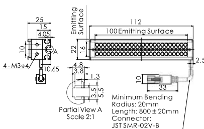
7.OPT-LI11222
