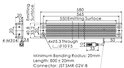
22.OPT-LI58041
