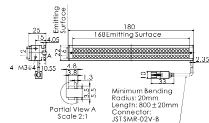
12.OPT-LI18022
